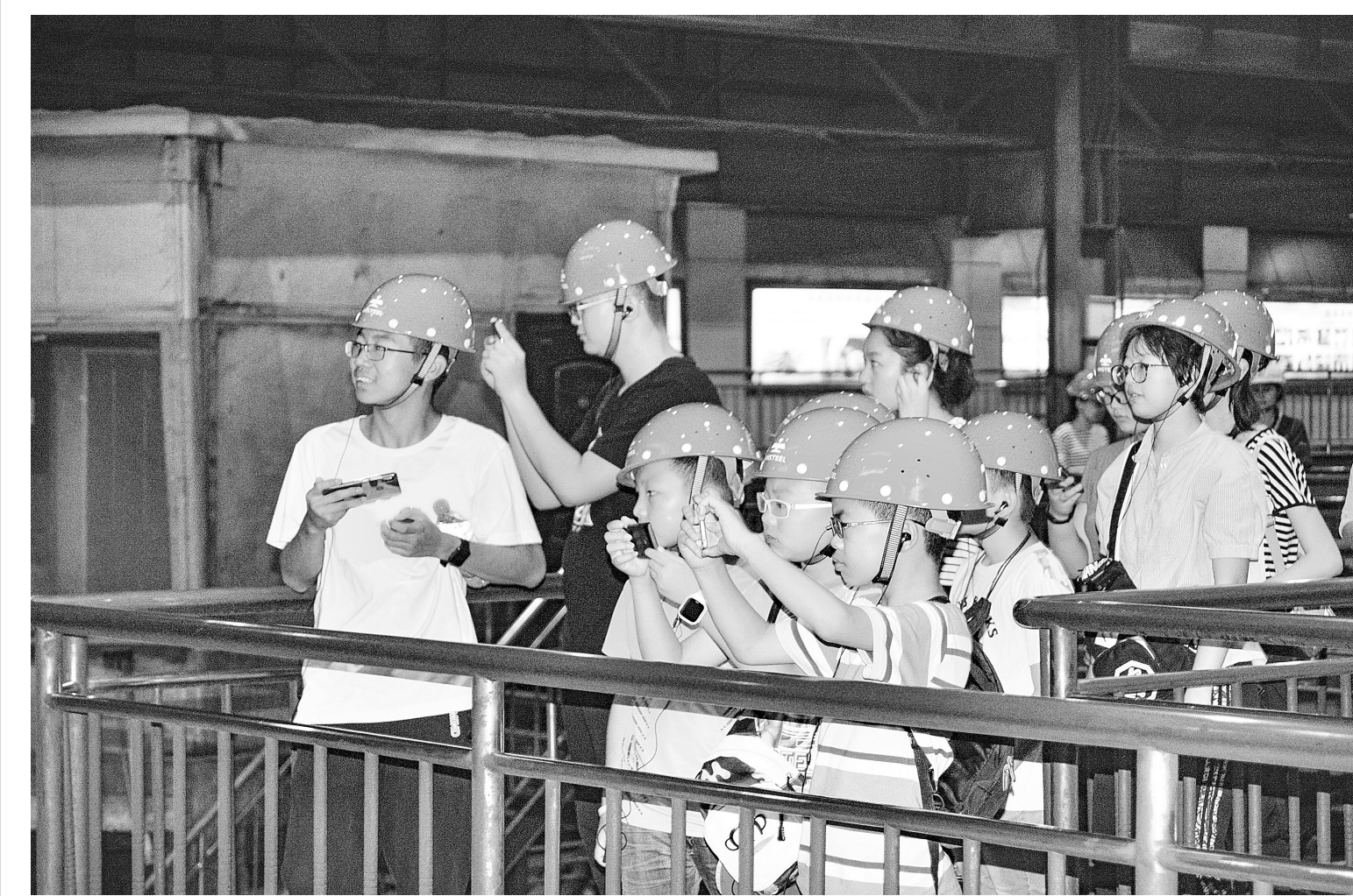
7月27日,35名攀钢职工子女走进了攀钢钒轨梁厂,参观了百米钢轨的生产全过程。孩子们看到钢坯通过加热炉,经多次“压面条”式的轧制,成为了百米钢轨,不断发出惊叹,并纷纷拍照,留下精彩的瞬间。这是攀钢集团有限公司举办的“职工子女走进新攀钢”系列活动中的一场,该活动旨在通过展示攀钢先进、创新、环保的新面貌和良好社会形象,让职工子女感知攀钢、关注攀钢,增强自豪感。 孟祥林 王训华 摄
