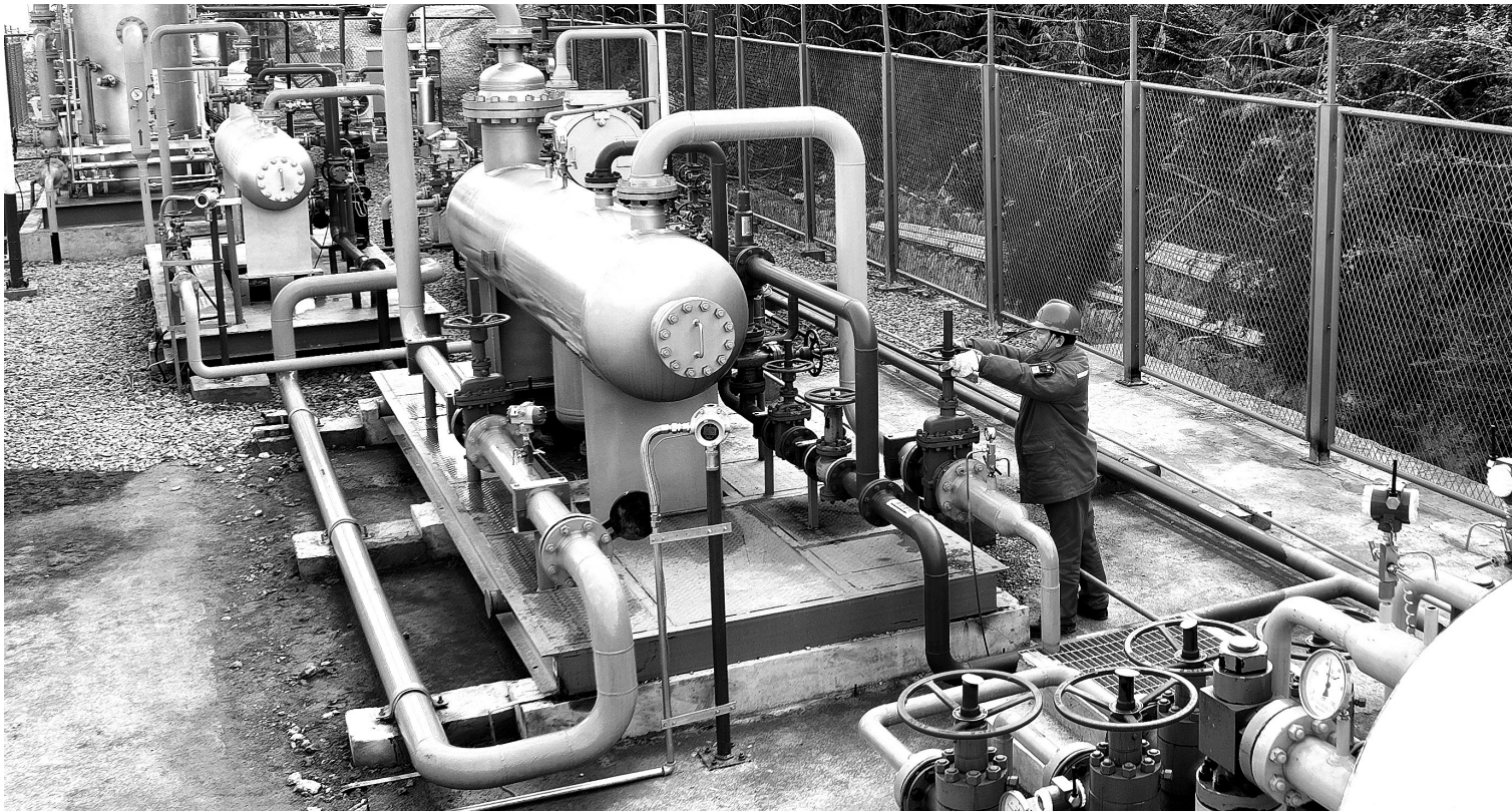
重庆市万盛经开区曾经因煤而兴、依煤而盛,如今成为全国资源型城市转型试点城市。近年来,万盛经开区推进关闭煤矿复绿复垦治理,推动资源型城市全面转型升级,发展页岩气产业,努力实现生态效益与经济效益的双赢。图为1月7日,位于万盛经开区南桐镇金龙村的当地第一口页岩气井平台新页1HF井平台向城镇燃气主管网输送页岩气。 曹永龙 摄
